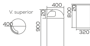
BASURERA 50 LT.
