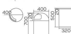
BASURERA 38 LT.
